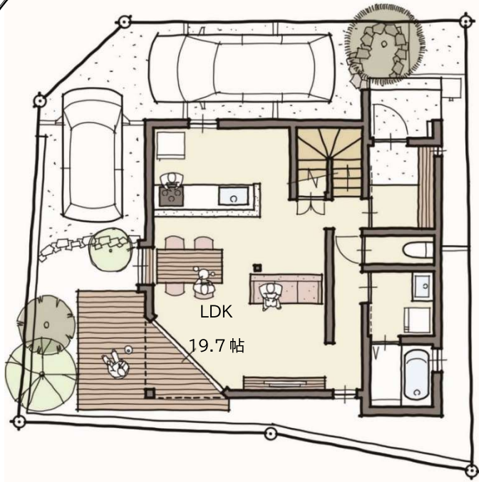
配置図・1階平面図
