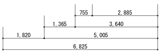
● 1階 平面図 S:1/100
