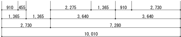
●1階 平面図 S:1/100
